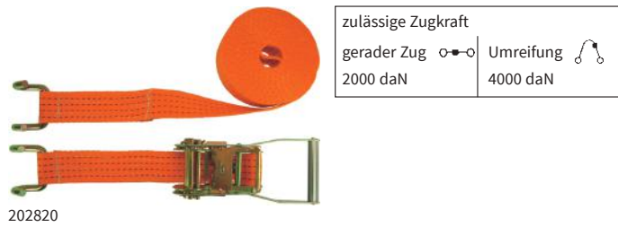
202820 Verzurrgurte BSN 2-teilig, Polyesterband, mit Ratsche, DIN EN 12 195-2, System 2000 daN, 50 mm
